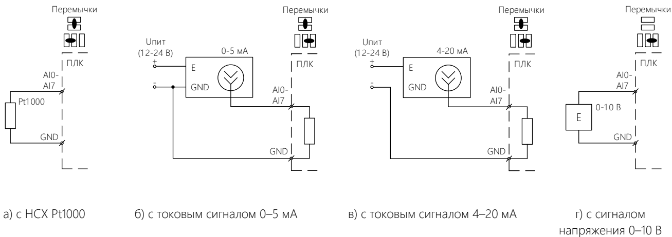
Рисунок 8. Подключение датчиков.
