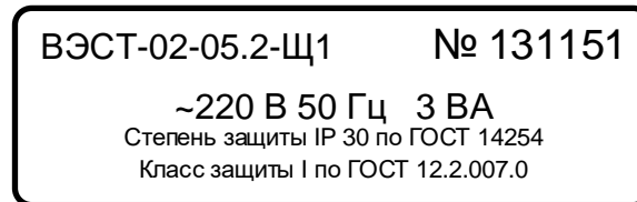
Рисунок 3. Пример маркировки прибора.
