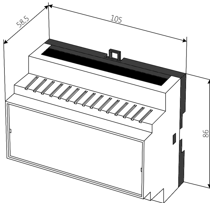
Рисунок 4. Габаритные размеры ВЭСТ-02.
