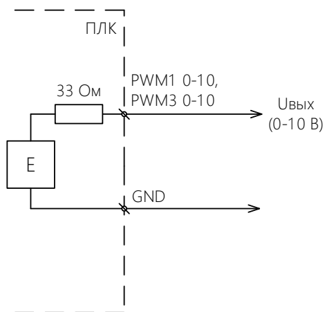
Рисунок 9. Подключение внешних устройств с управлением сигналом напряжения 0–10 В.
