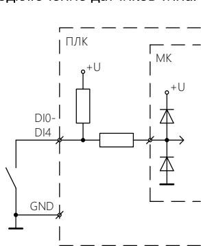
а) «сухой контакт»
