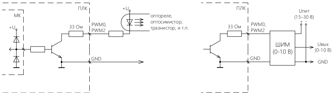
а) транзисторный «открытый коллектор»
