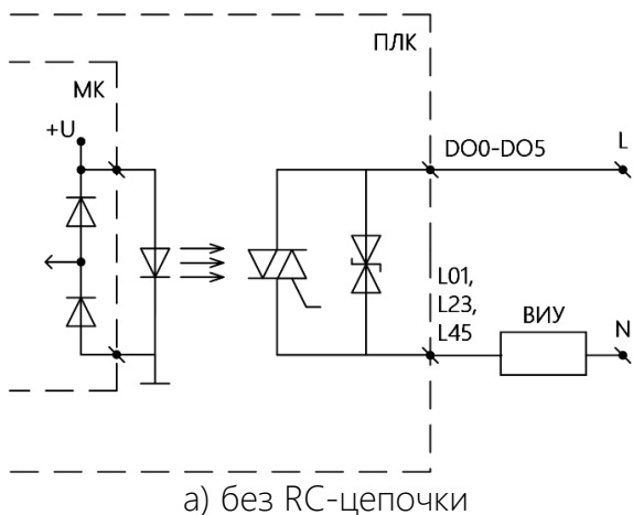
Рисунок 9 – Подключение внешних устройств к дискретным симисторным выходам
