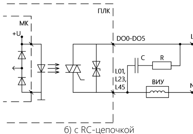
Рисунок 9 – Подключение внешних устройств к дискретным симисторным выходам
