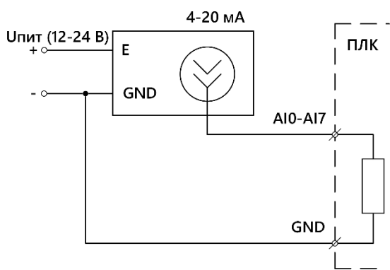
в) с токовым сигналом 4-20 мА
