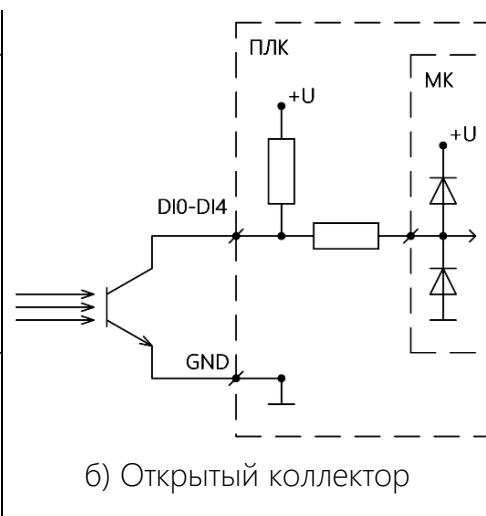
Рисунок 8 – Подключение датчиков
