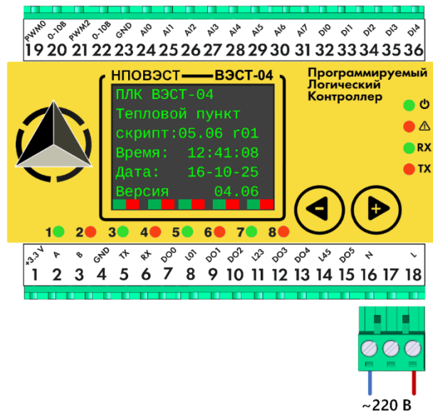
Рисунок 13 – Подключение питания
