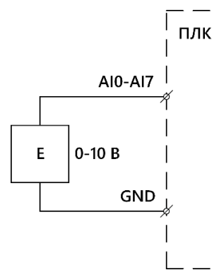
г) с сигналом напряжения 0-10 В
