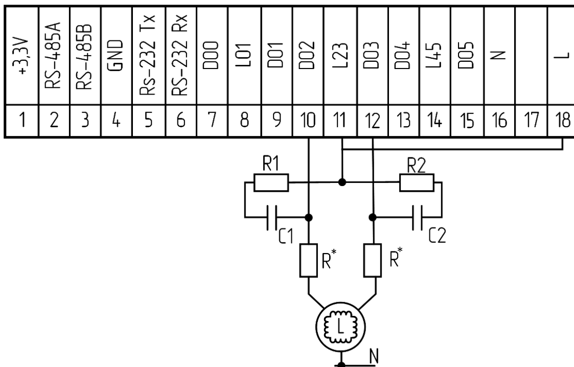
Рисунок 14 – Подключение RC-цепочек
