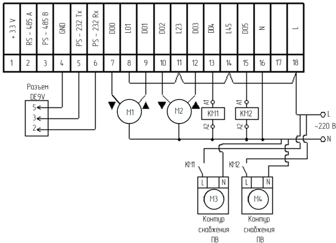
Рисунок Б.2 – Схема подключения нижней клеммной колодки
