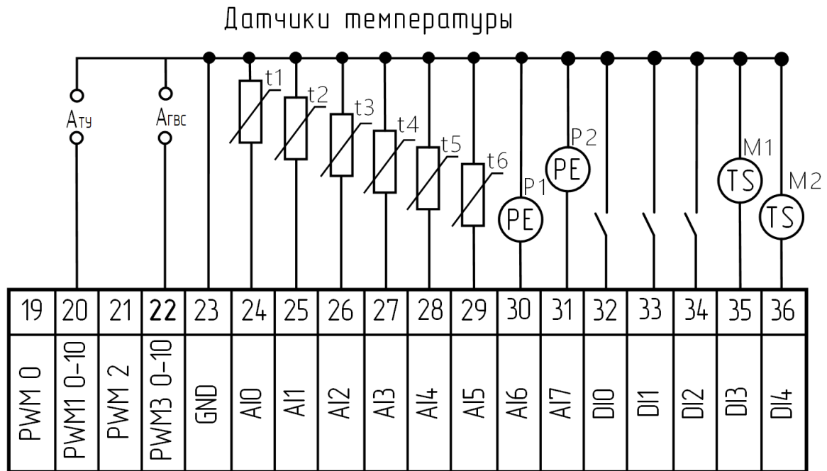
Рисунок Б.1 – Схема подключения верхней клеммной колодки
