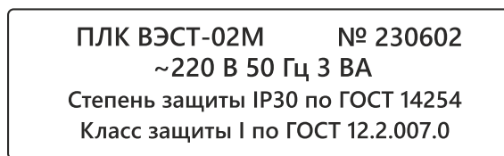
Рисунок 11. Пример маркировки прибора
