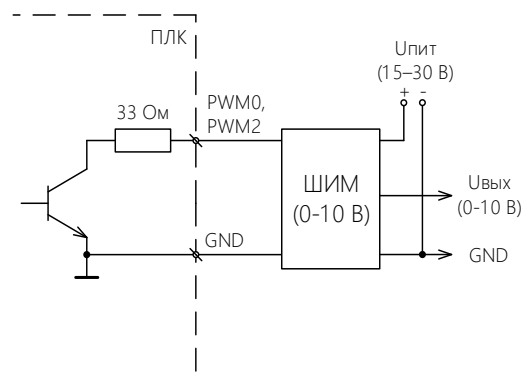
б) ШИМ
