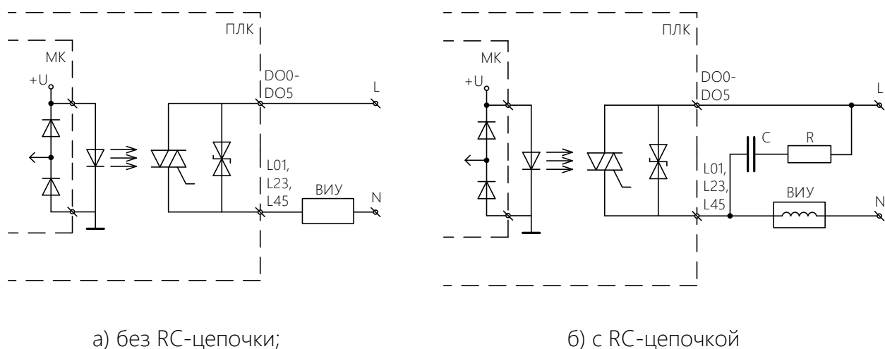
Рисунок В3. Подключение внешних устройств к дискретным симисторным выходам
