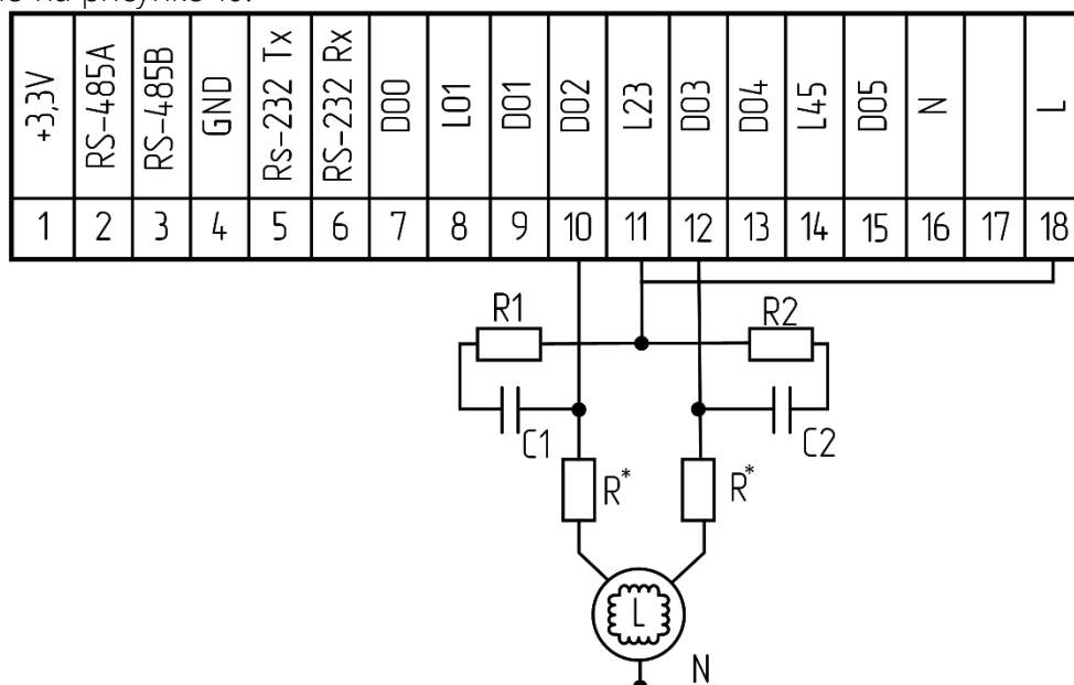
Рисунок 10 – Подключение RC-цепочек
