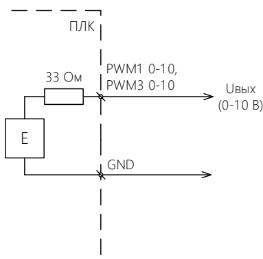
Рисунок В13. Подключение внешних устройств с управлением сигналом напряжения 0–10 В
