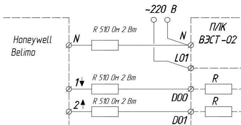
Рисунок 9 – Рекомендация по подключению приводов
