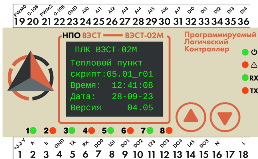
Рисунок 1 – Лицевая панель ПЛК ВЭСТ-02М
