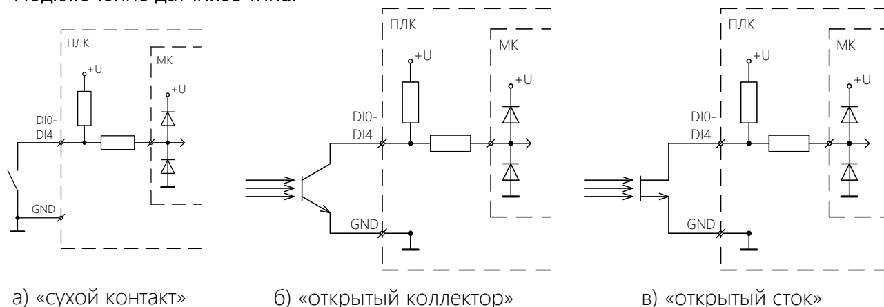
Рисунок В2. Подключение датчиков
