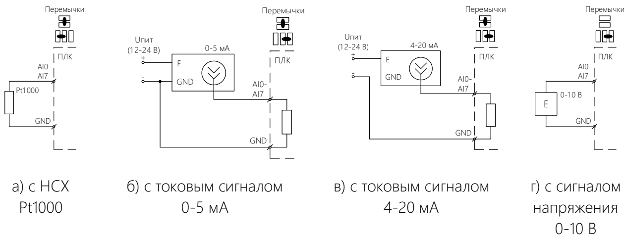
Рисунок В12. Подключение датчиков
