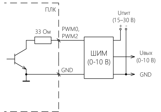
б) ШИМ
