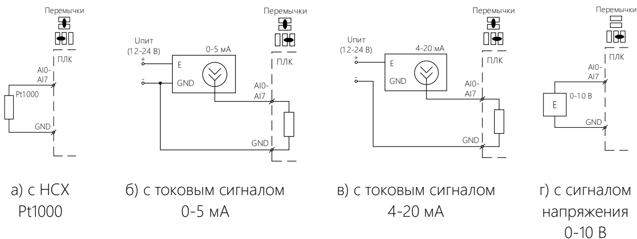
Рисунок В4. Подключение датчиков
