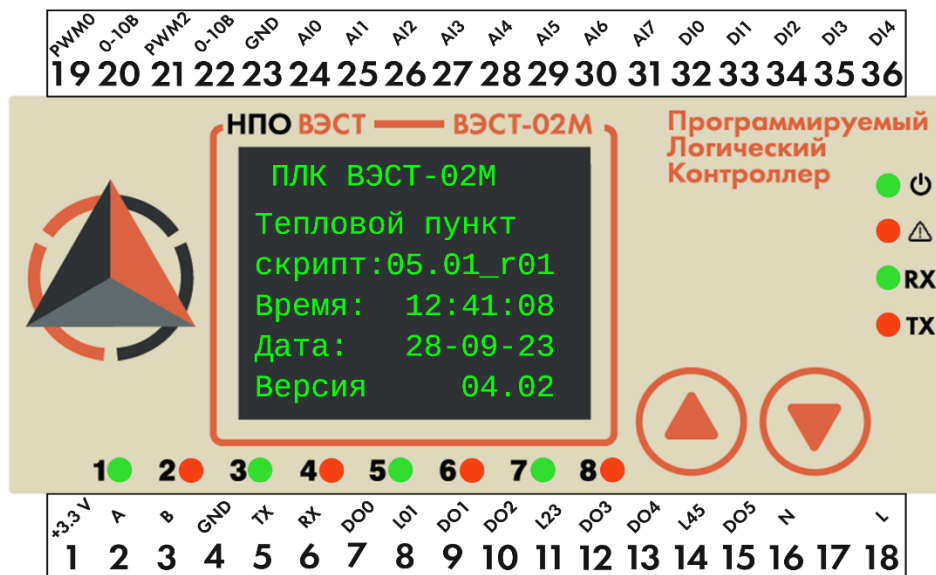
Рисунок 1 – Лицевая панель ПЛК ВЭСТ-02М
