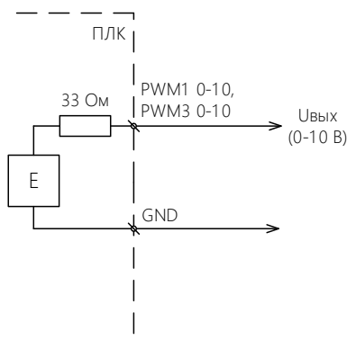
Рисунок В5. Подключение внешних устройств с управлением сигналом напряжения 0–10 В
