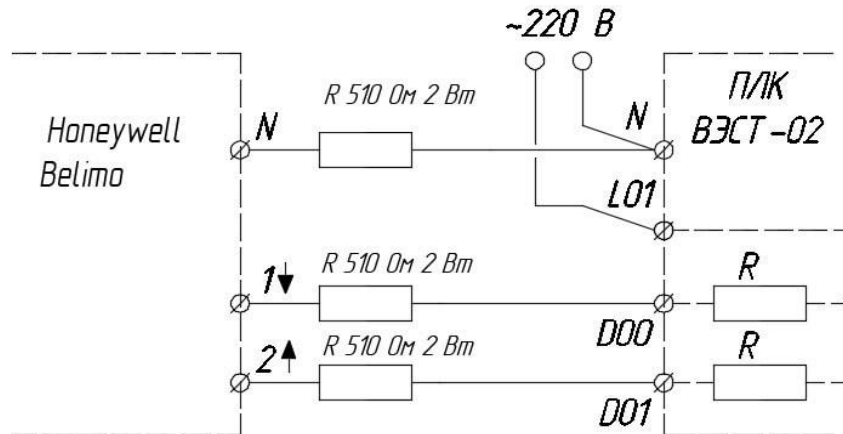
Рисунок 2 – Рекомендация по подключению приводов
